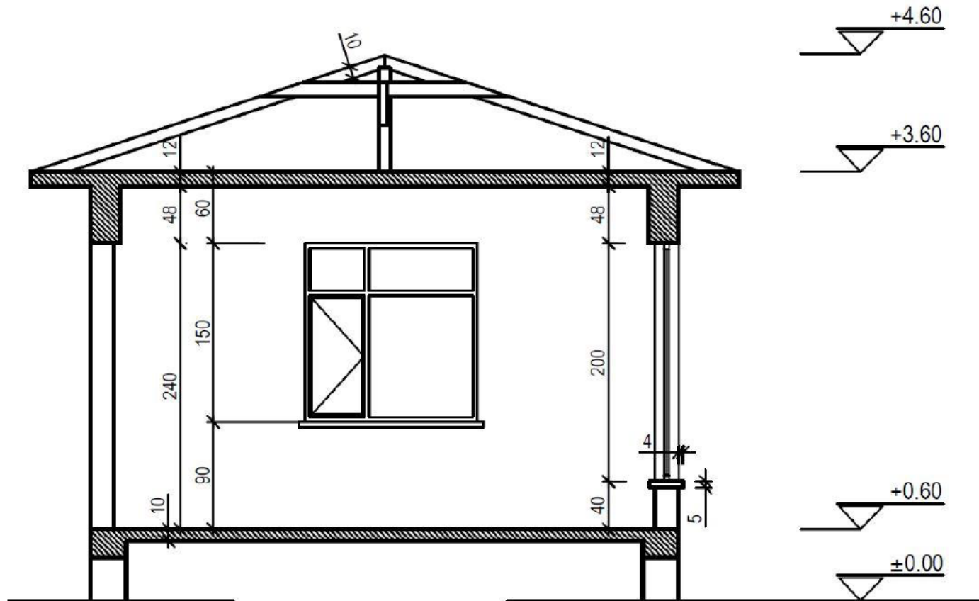
B-B KESİTİ
