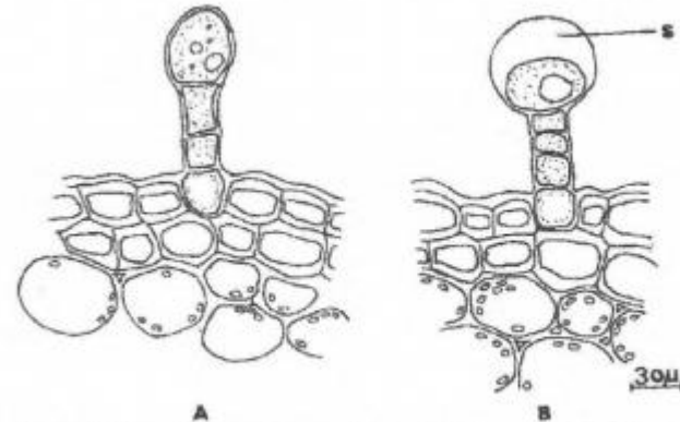
2.30. Sardunya ( Pelargonium zonale ) yaprak sapından alınan enine kesitte salgı tüyü: A, genç tüyü; B, salgı depolanmış tüy; S, salgı.
