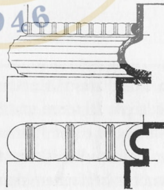
62 Delphi, Apollon-Heiligtum. Wandfußprofile der Schatzhäuser von Knidos und Siphnos
