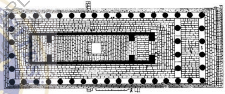
231 Selinus, Akropolis. Tempel C. Grundriß (1 : 800)
