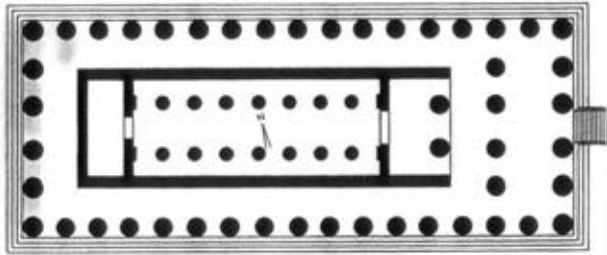
218 Syrakus, Apollon-Tempel. Grundriß (1:800)
