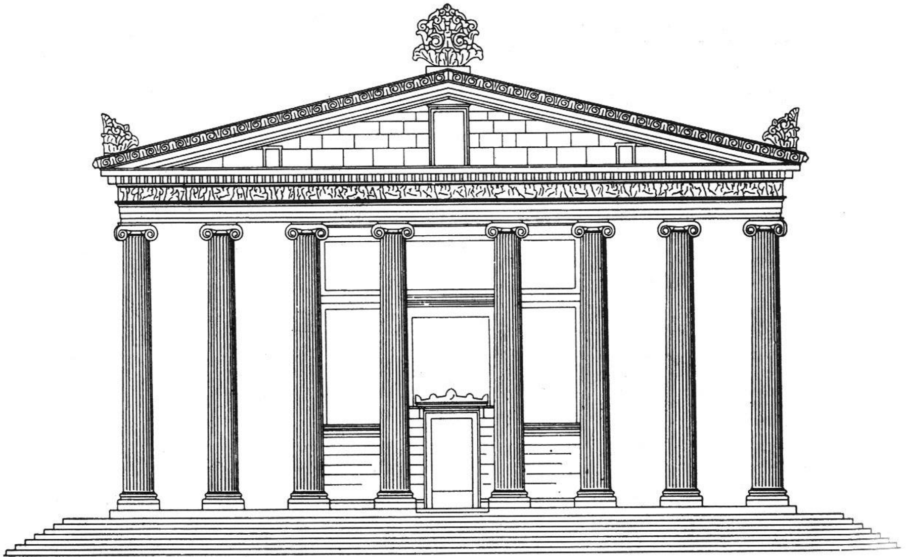
321 Magnesia am Mäander, Tempel der Artemis Leukophryene. Westfront (1 : 400)
