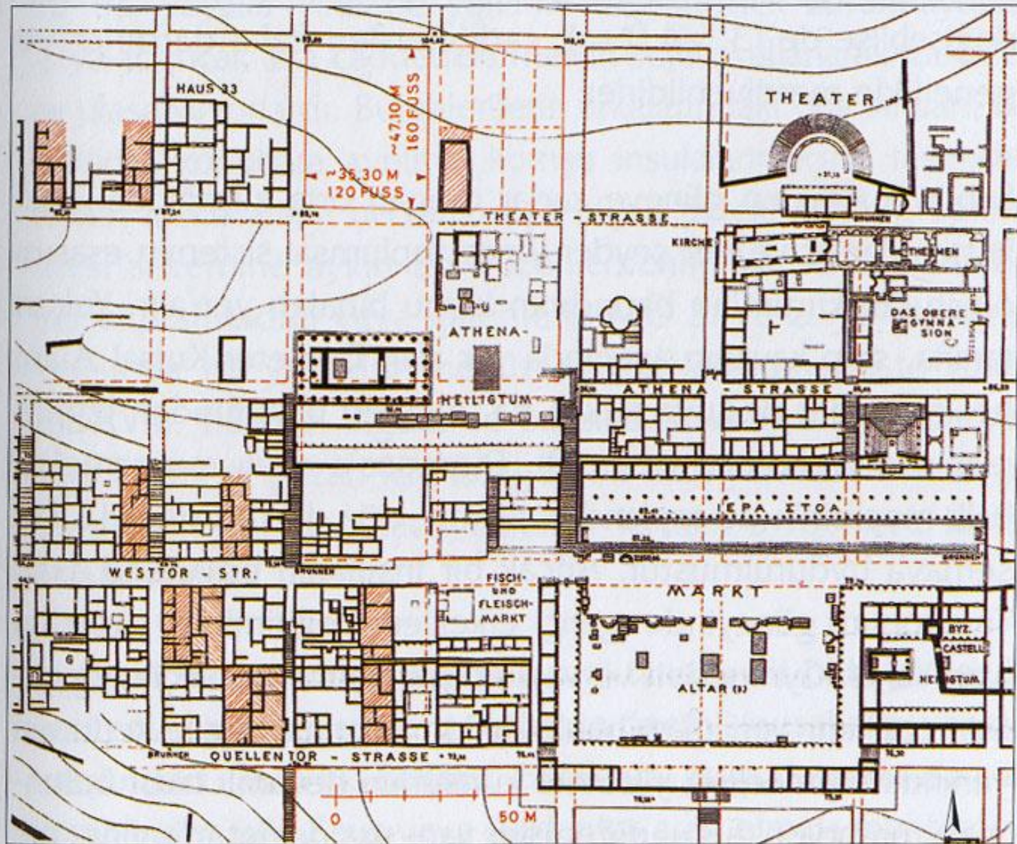
Res. 21 Şehrin orta kısmının ölçekli planı.
