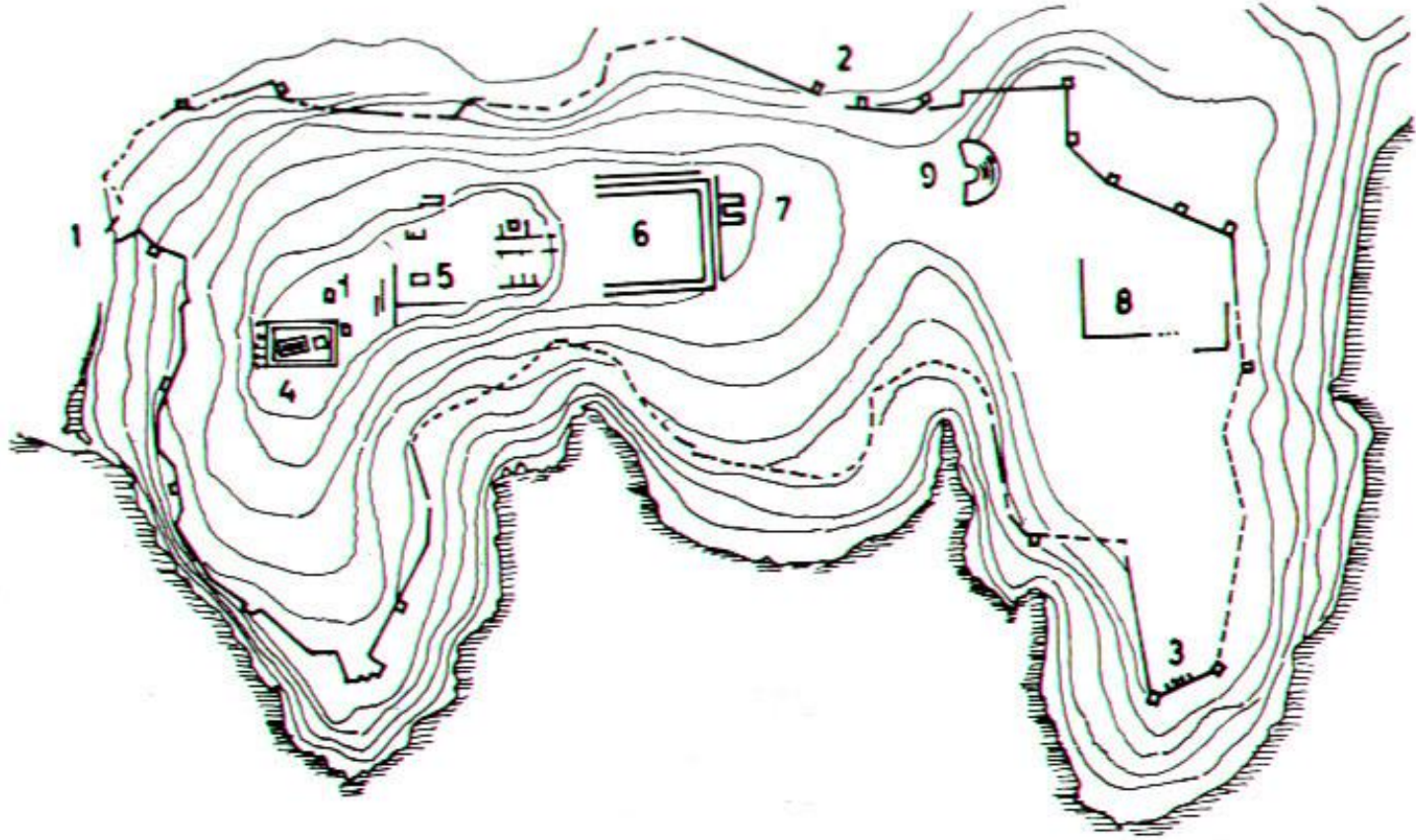
Şekil 312 Notion'un Planı. Hellenistik Dönem'de inşa edilmiş olan kent duvarının günümüze değin kalmış olan üç girişi bulunmaktadır. 1) Batı Kapısı. 2) Kuzey Kapısı. 3) Güneydoğudaki merdivenli giriş. 4) Hadrian Dönemine (M.S. 117-138) tarihlene Athena Kutsal Yeri. Etrafını çeviren Dor düzenindeki stoklarla, Korinth düzenindeki bir templum in antisin temelleri. 5) Başka bir tapınağın kalıntıları. 6) Merkezi Agora. 7) Bouleuterion. 8) Doğu agora. 9) Hellenistik Dönem'de inşa edilip, Roma Çağı'nda değişikliğe uğrayan tiyatro.
