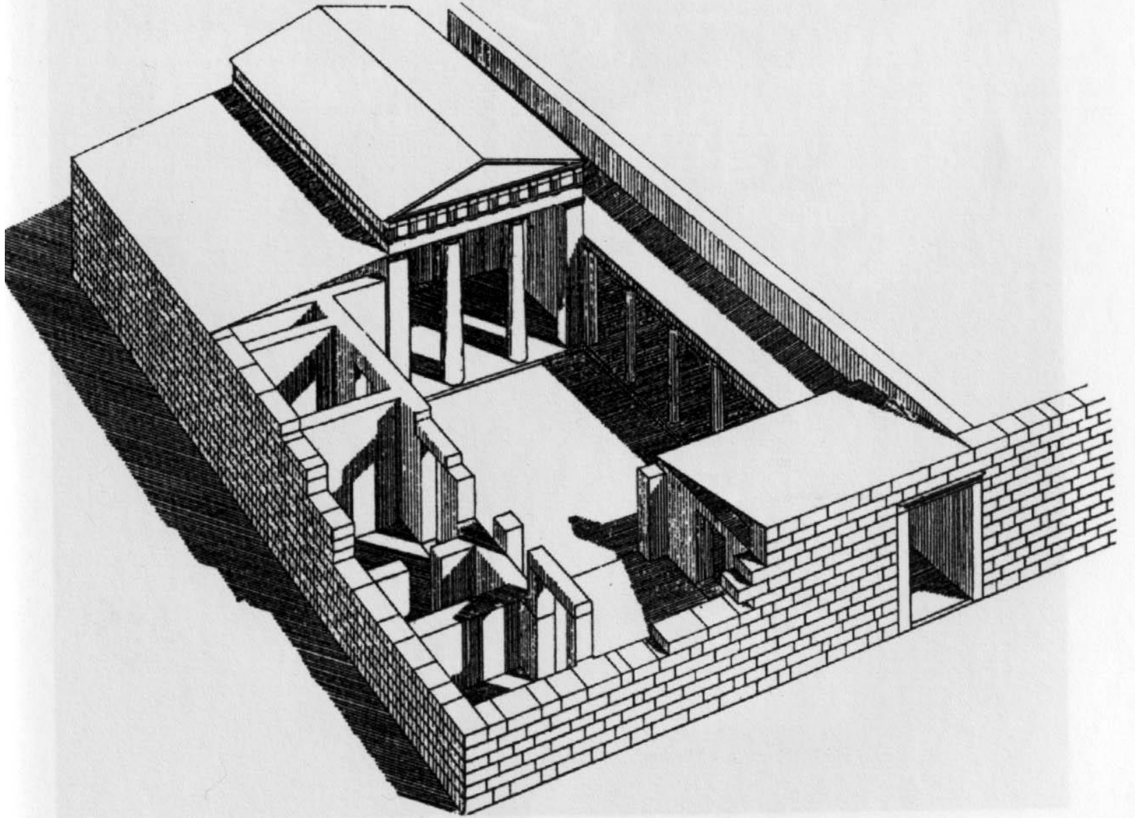
Res. 130 33 no'lu batı evi. Güneybatıdan 1. evredeki görünüşün rekonstrüksiyonu.
