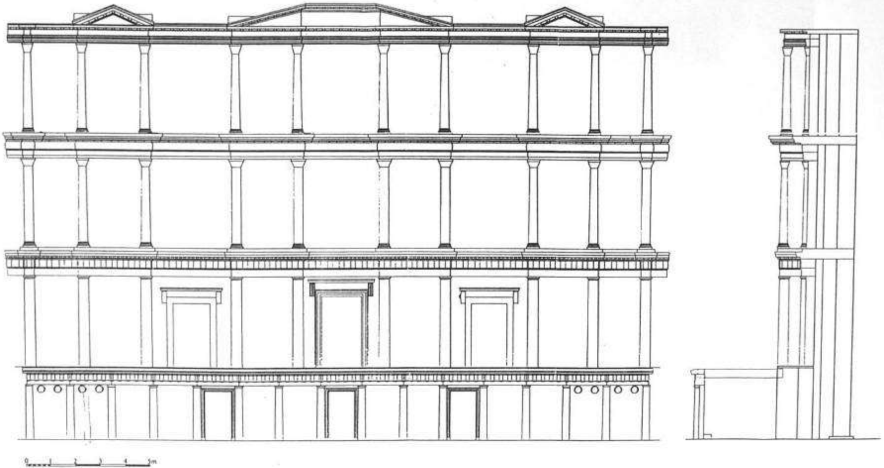
Rekonstruktion der scaenae frons des Theaters von Stratonikeia (nach I.H. Mert [1998] Abb. 18)
