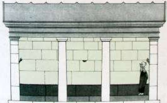
Res. 89 Rekonstrüksiyon: Plan ve ön cephe (1. Evre)
