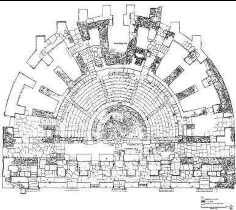
Fig. 16. Plan of Bouleuterion
