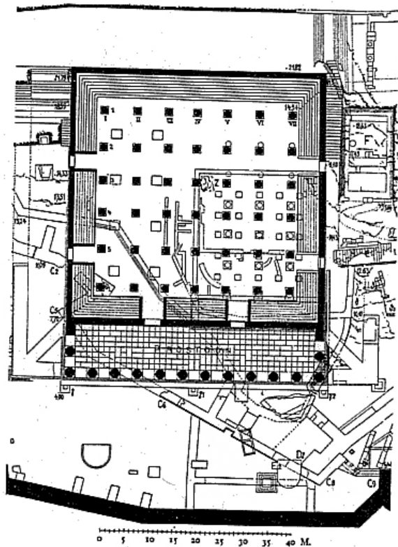
Fig. 74. Telesterion, Eleusis; planta general de los restos subsistentes (el norte a la derecha, aproximadamente)
