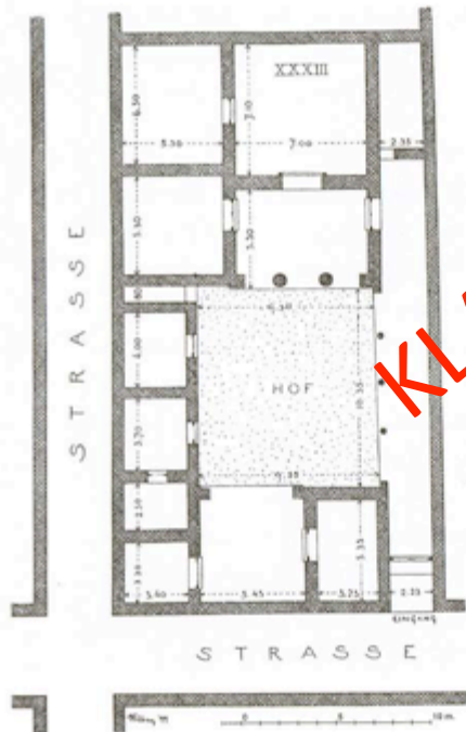
Abb. 129 Haus 33 West. Prostaion-Grundriß der 1. Phase
