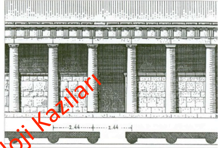
Abb. 62 Südhalle der Agora. Rekonstruierte Ansicht der mittleren Nordfront mit Wand zwischen den Säulen
