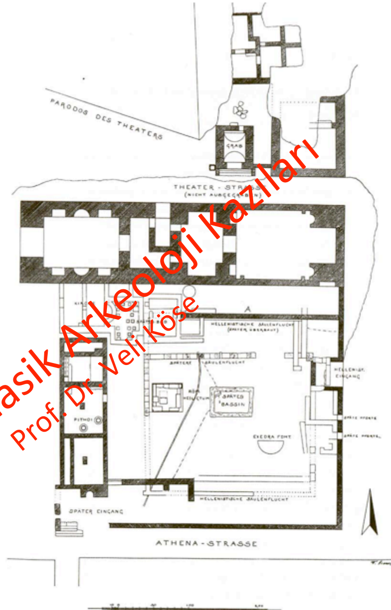
Abb. 160 Übersichtplan oberes Gymnasion, Thermen und Heroon
