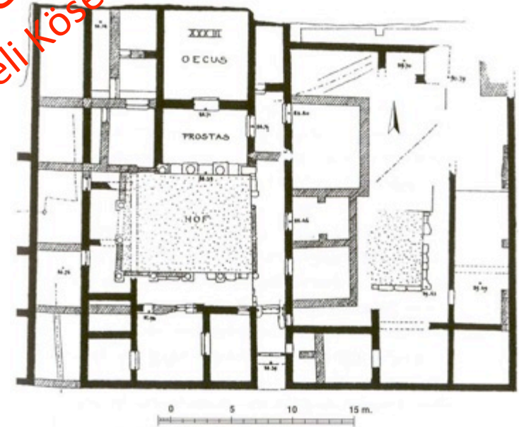
bb. 124 Haus 33. Grundriß mit Phase 1 (schwarz) und 2 (schraffiert)
