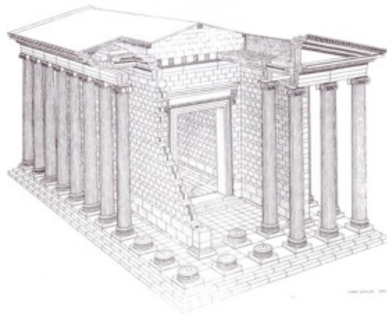
Abb. 97 Athena-Tempel. Isometrische Rekonstruktion der Südostansicht
