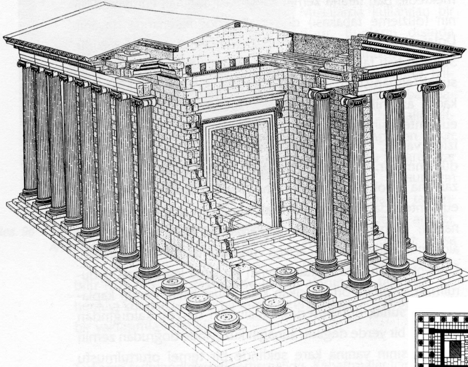
Res. 97 Athena Tapınađı. Güneydođudan görünüşünün isometrik rekonstrüksiyonu.
