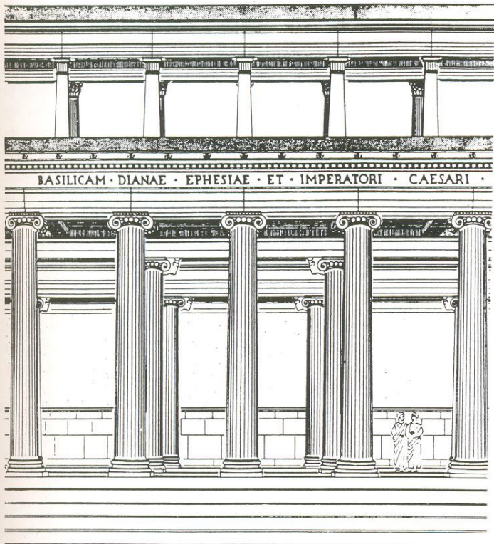
Fig. 293: Façade restituée de la basilique d'Ephèse, d'après E. A. Fossel-Peschl.
