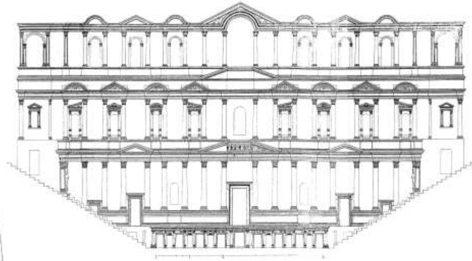
Rekonstruktion der scenae frons des Theaters von Perge (nach A. Öntürk [2000] Taf. 4)
