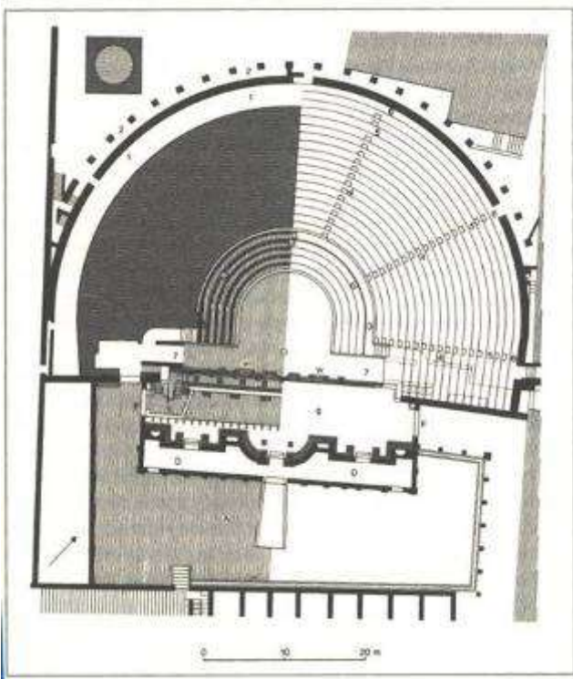
Roma-İmparatorluk tipi scaenae frons, Pompeii Tiyatrosu
