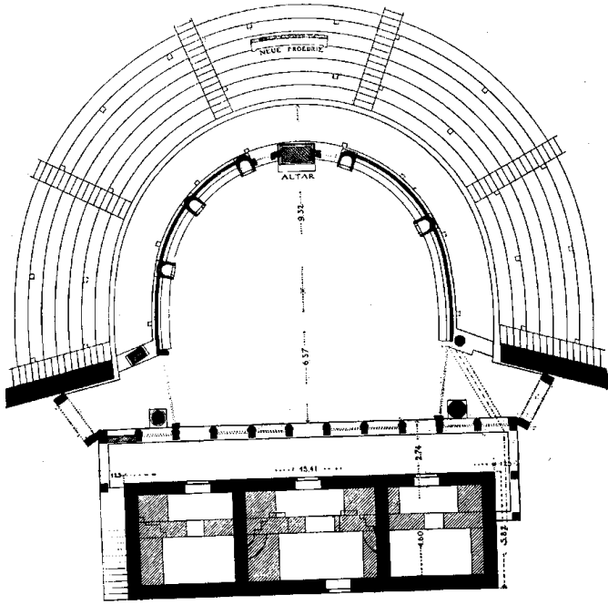
Şek. 343 - Priene. Tiyatro. Yapı planı (bkz. Şek. 344).
