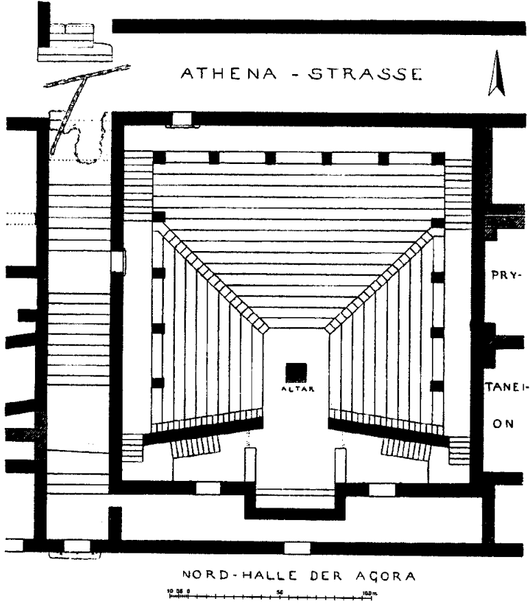
Res. 39 Bouleuterion. Plan (I. evre).
