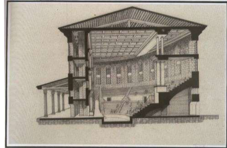
27. Odeon'un bayuna kesitini gösteren rekonstrüksiyon çizimi. Dr. G. Izeneur.
