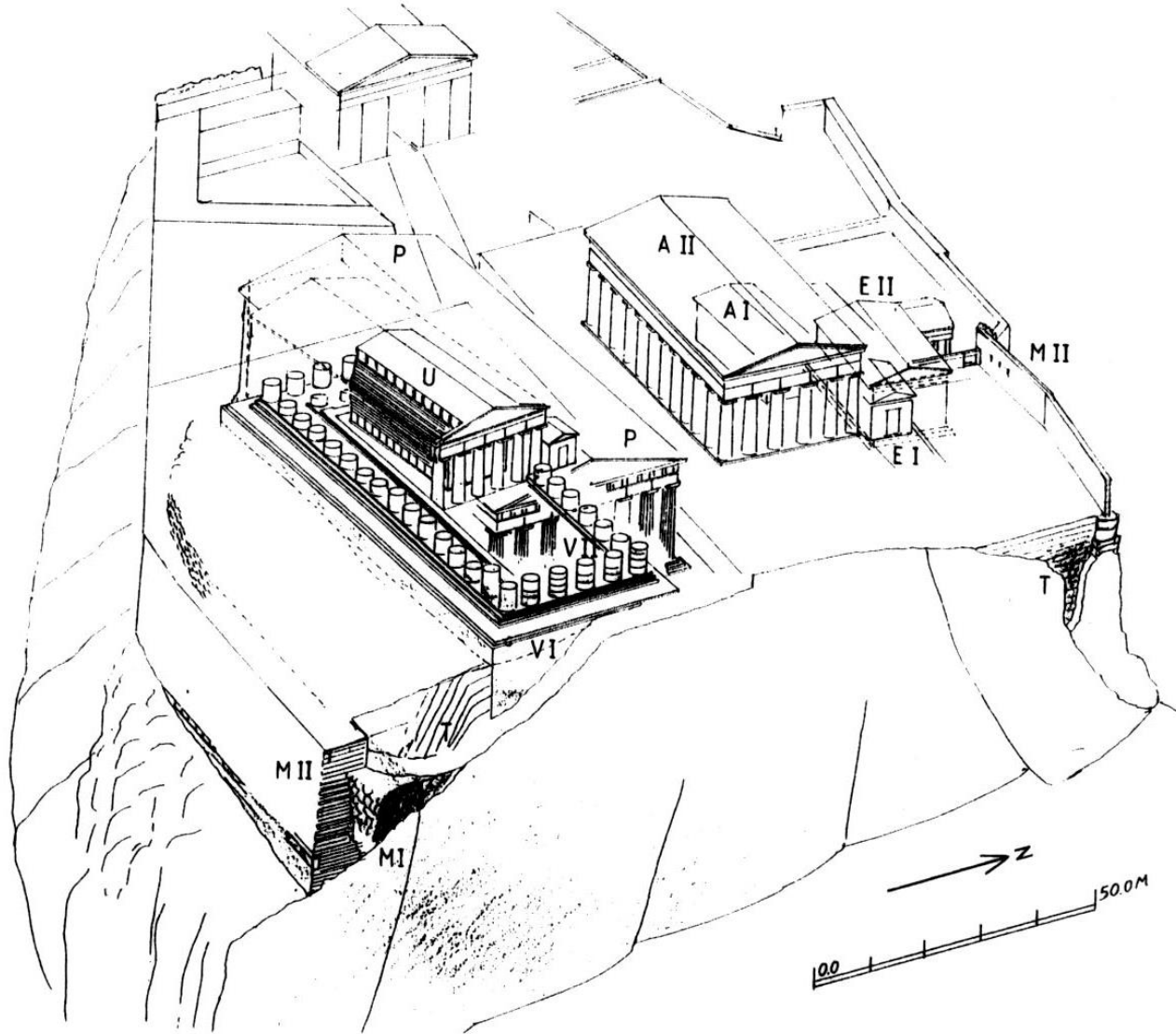
132 Die Bauphasen der Athena-Tempel (nach M. Korres): U Urparthenon (Poros. Anfang 6. Jh.); V I Vorparthenon I (Poros. Um 510, unfertig); V II Vorparthenon II (Marmor. Nach 490, unfertig); P Parthenon (447); A I ältester Athena-Tempel. Anfang 7. Jh.; A II dessen Nachfolger, der »Alte Tempel« (520/500); E I Erechtheion I. Naiskos (Anfang 5. Jh.?); E II Erechtheion II (~ 421 – 406); M I mykenische Mauer; M II klassische Mauer; T Tyrannen- und Perserschutt
