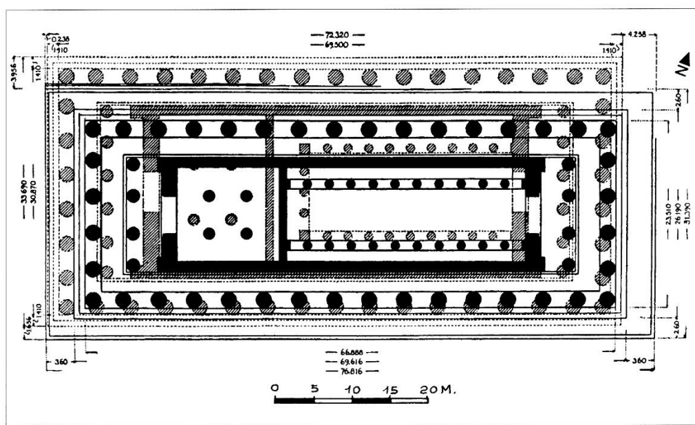
Fig. 101. Athènes, Acropole. Plans superposés du Pré-Parthénon (en noir) et du Parthénon (en gris). D'après B. H. Hill, AJA 1912, pl. 9.
