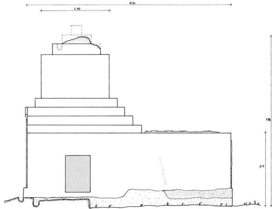
ESKI FOÇA TAŞ KULE SIDE ELEVATION
