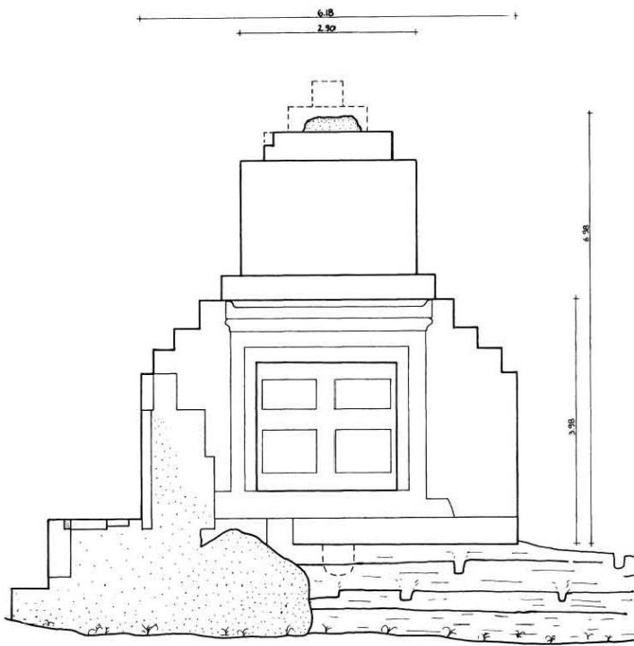
ESKI FOÇA TAŞ KULE FRONT ELEVATION
