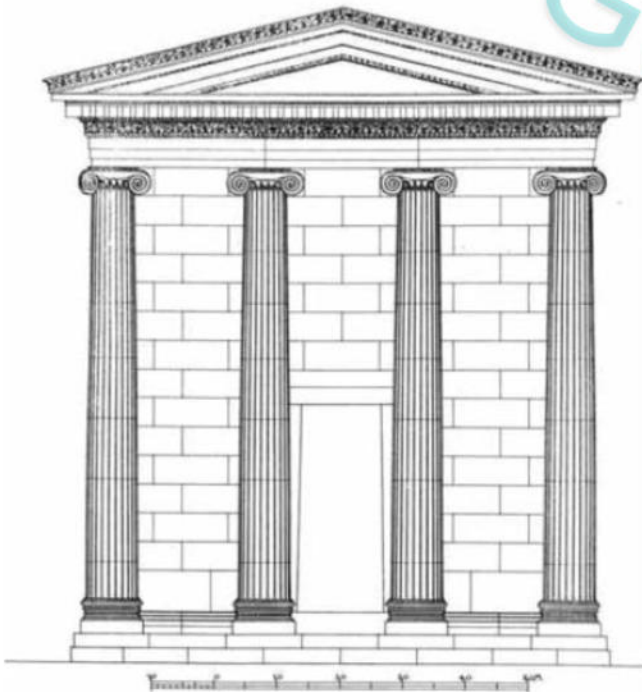
Abb. 135. Ansicht des Naiskos, Rekonstruktion von H. Knackfuss (Z. 597).
