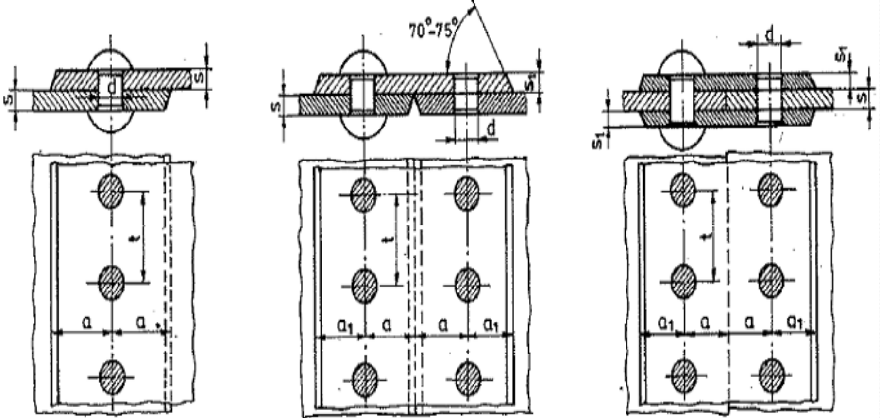
Tek sıralı bindirme perçinleme.
