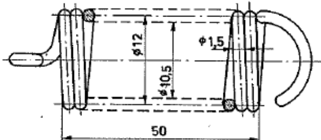
ÇEKME YAYI
