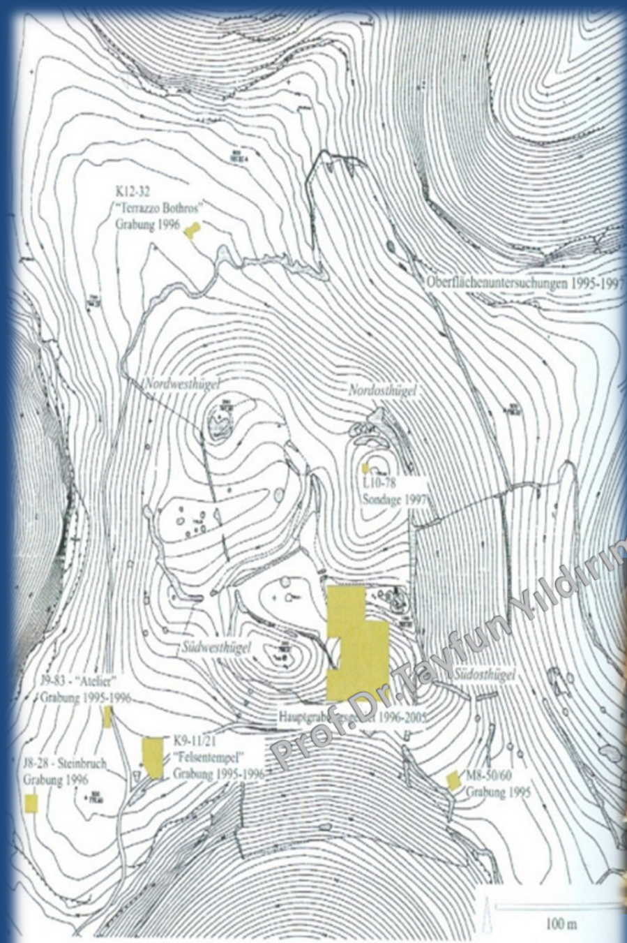
Resim 31: Göbekli Tepe'nin topografik planı.
