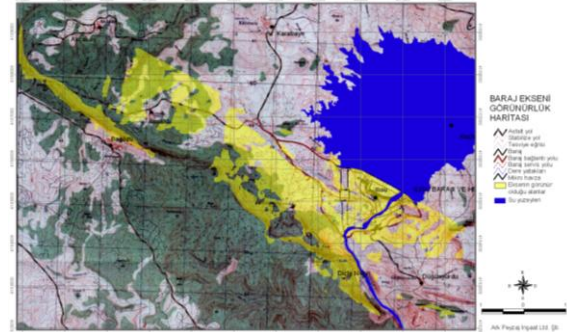
Şekil 4. İhsu HES barajı kret bölgesi görünürlük analizi
