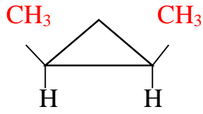
Cis-1,2-dimetilsiklopropan
