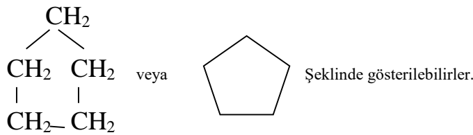
Siklopentan
