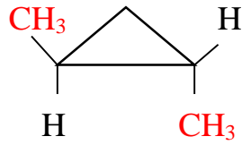
Trans-1,2-dimetilsiklopropan
