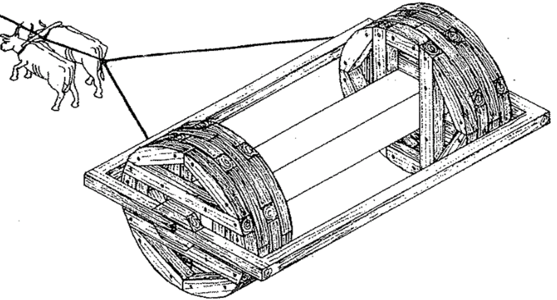
. Metagenes'in metoduna göre blokların taşınması (Coulton, Architects Fig. 62).
