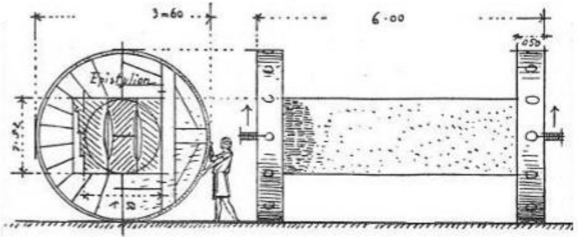
Resim 12. Taşa ahşap bir tekerlek giydirilerek taşınması (Orlandos 1968, 26, Fig. 10)
