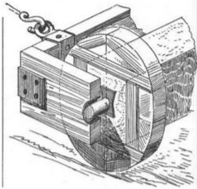
Taşa ahşap bir tekerlek giydirilerek taşınması (Orlandos 196
