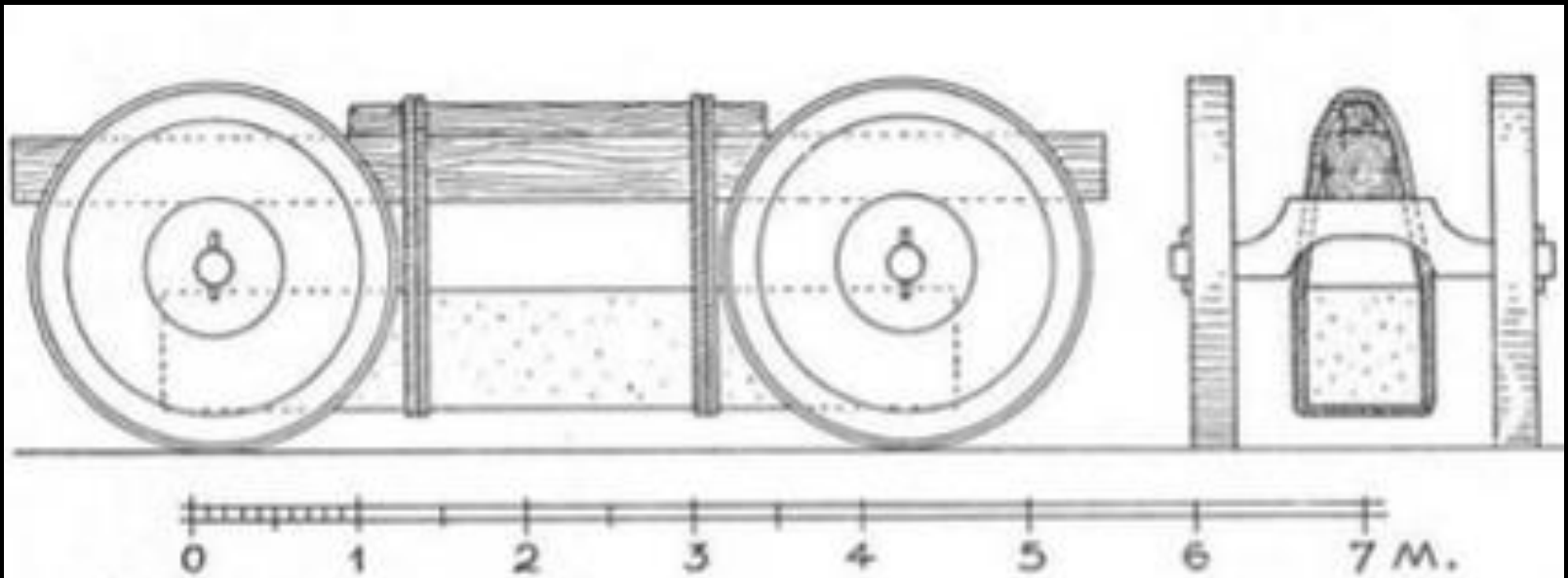
Resim 14. Taşa ahşap bir tekerlek giydirilerek taşınması (Orlandos 1968, 28, Fig. 13)
