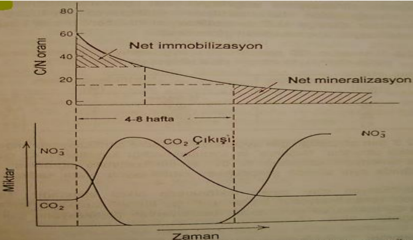
Şekil 12.3. Düşük düzeyde N içeren (C/N oranı yüksek) bir organik materyalin parçalanması esnasında topraktaki \text{NO}_3 azotunun değişimi (Tisdale ve Nelson, 1993).
