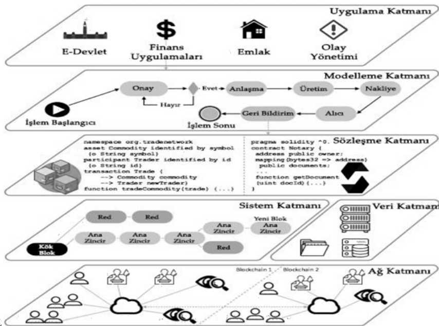
Şekil 2. Blokzincir Katmanları
