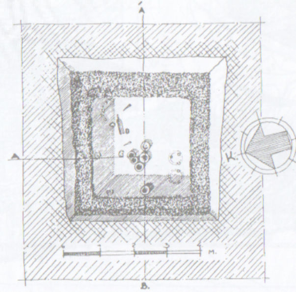
MEZAR ODASI PLANI
