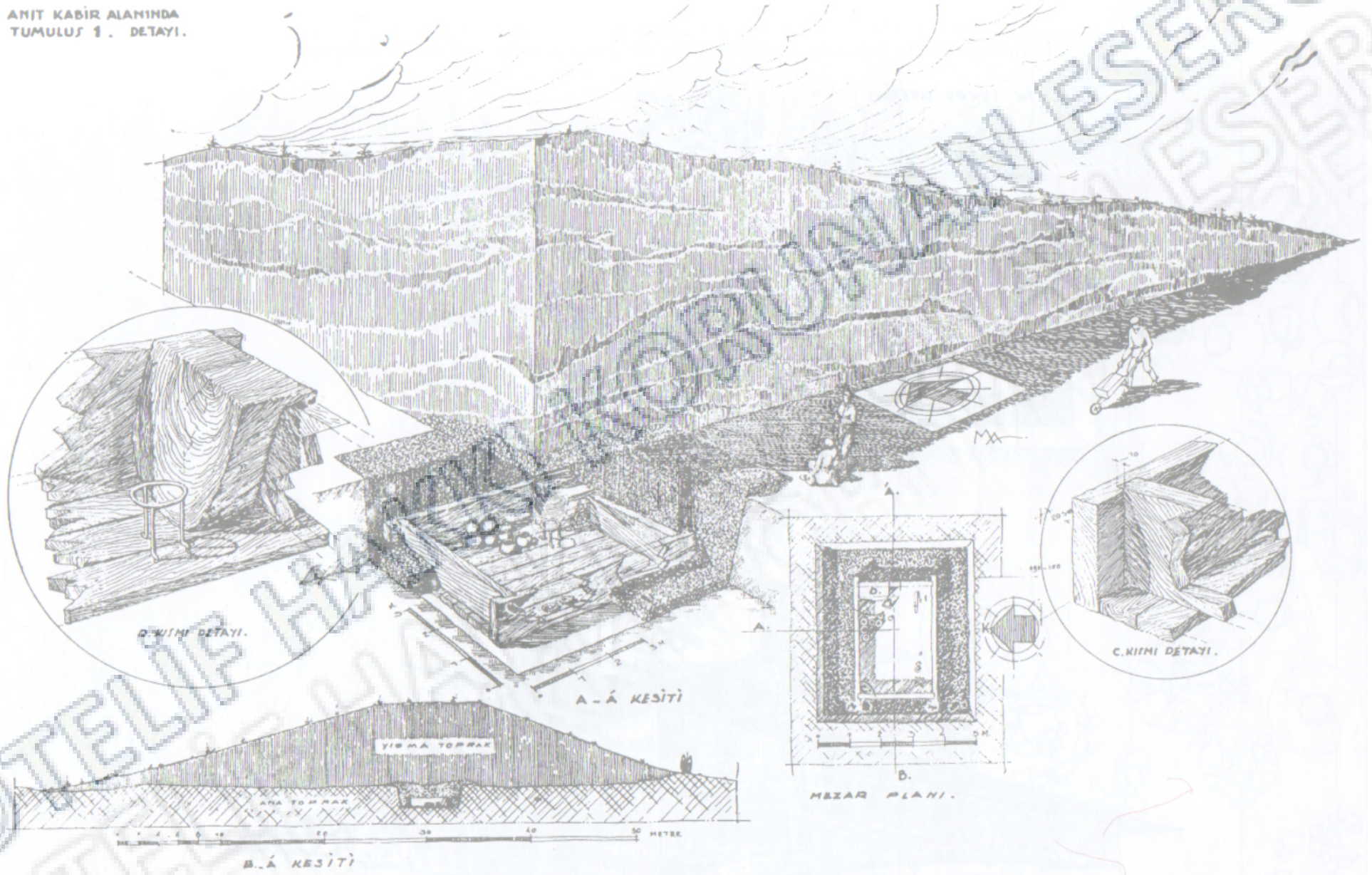
Ankara Anıtkabir Alanında Kazılan Phryg Tümülüsü I'nin Ayrıntılı Plân ve Kesitleri (T. Özgüç, Anıtkabir Tümülüsleri Kazısı; Belleten XI, Ankara 1946).
