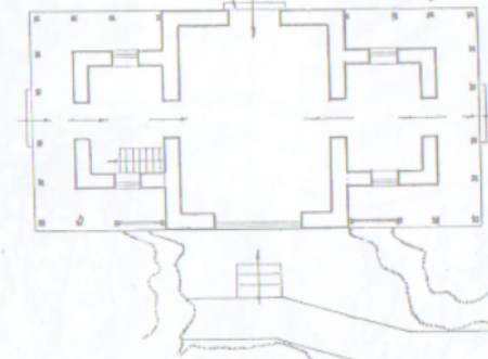
2. ZEMİN KAT PLANI 2. Plan.- Rez-de-chaussée
