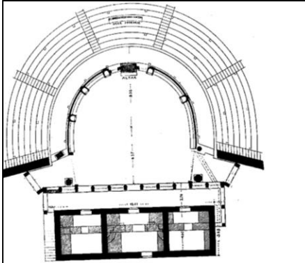
Şek. 343 - Priene, Tiyatro. Yapı planı (bkz. Şek. 344).
