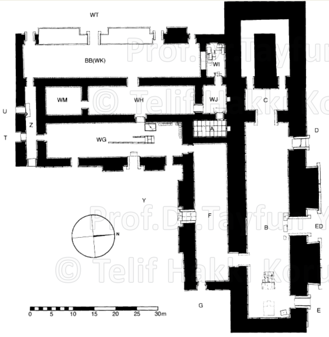
Kuzeybatı Sarayı Taht odası ve özel salonlar (F,G,H) Paley/Sobolewski 1987, plan 2.
