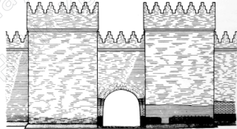
Fig. 92. Plan, elevation and reconstruction of the west gate. Batı Kapısı
