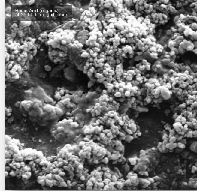
Humik maddeler
