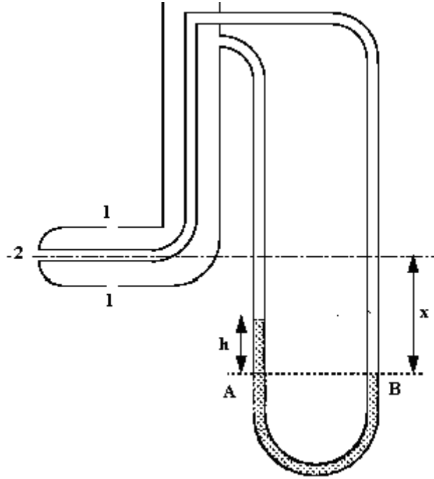
Şekil 3.3. Statik pitot tüpü (Edis 1972b, Sleight 2001, Hewakandamby 2012)
