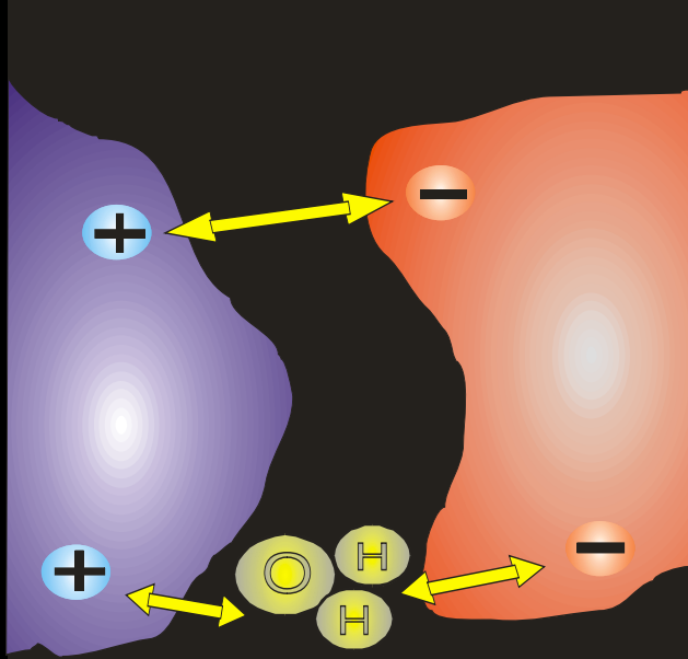
İyonik bağ
