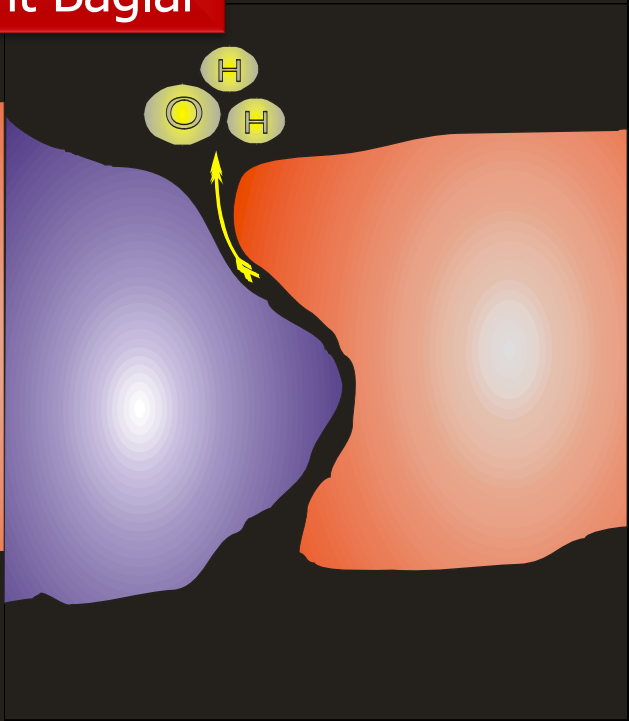
Hidrofobik bağ
