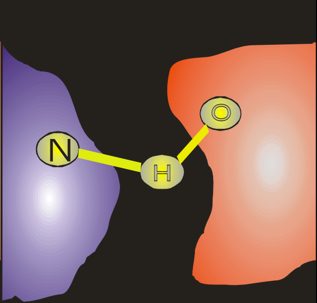
Hidrojen bağı
