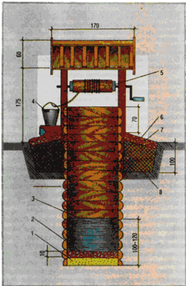
Рис. 1—48. Шахтный колодец, выполненный в виде деревянного сруба: грузом для опрокидывания; 5 — ворот; 6 — от- мостка; 7 — щебень; 8 — глиняный замок.
