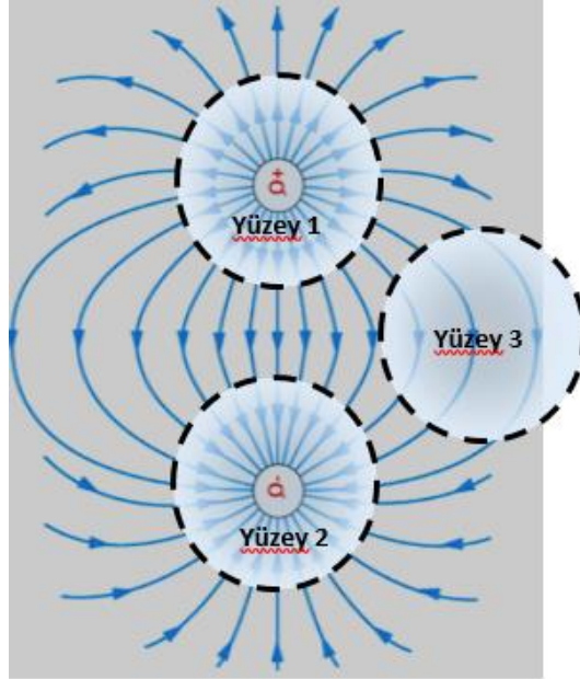
Şekil 3.3 Gauss Yüzeyi
