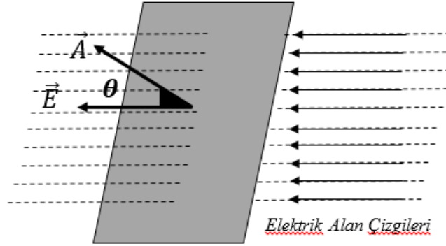
Şekil 3.1 Elektrik Akısı
