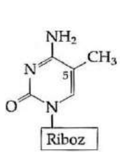
5-Metilsitidin
