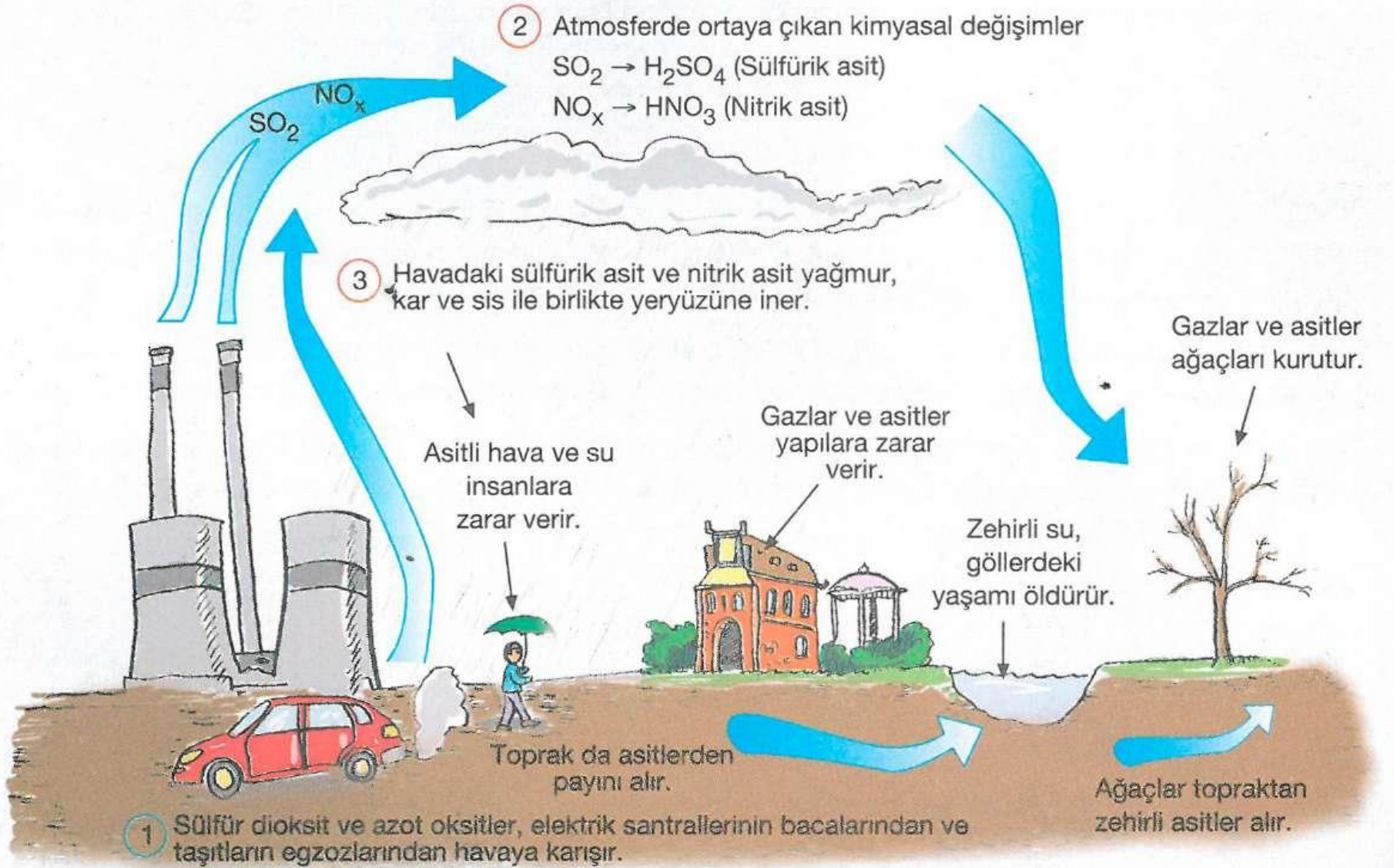
Şekil 3.1.8 Asit yağmuru
