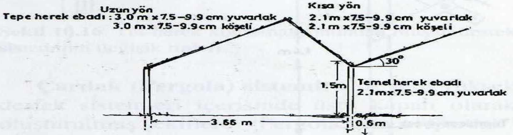
Şekil 10.25. Testere dişi çatılı çardak sistemi.
