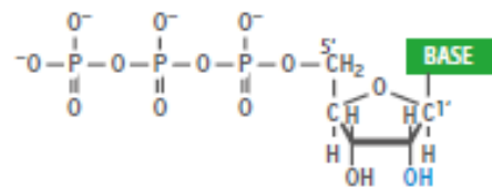
(B) Uracil
