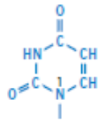
(B) Uracil
