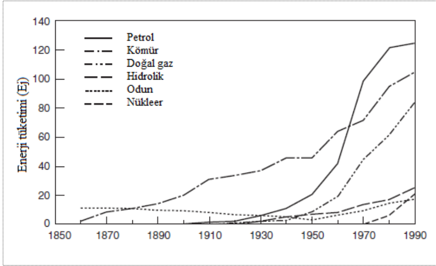
Dünya enerji tüketimi, 1850–1990 Kaynak: Weyant ve Yanigisawa, 1998: 208
