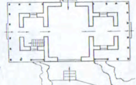
2. ZEMİN KAT PLAN 2. Plan - Rez-de-Chaussée
