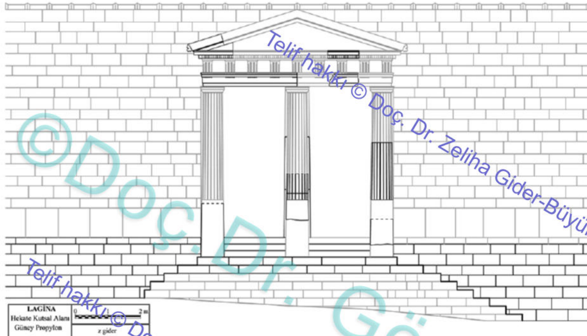
Fig. 7. Güney Propylon'un Ön Cephe Restitüsyonu
