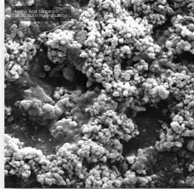
Humik maddeler
