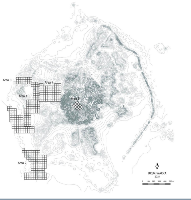
URUK KENTİNİN EN SON PLANI (MAGNOMETRİK) 2018
