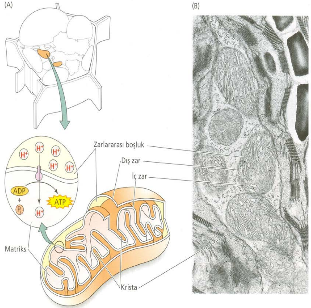
ŞEKİL 1.15 (A) İç zarlarda ATP sentezinde yer alan H^+ -ATPazların yerleşimleri dahil, bir mitokondrinin şematik görünümü. (B) Bermuda çimi ( Cynodon dactylon )'nin bir yaprak hücresinde bir mitokondrinin elektron mikroskopundaki görünümü (26.000x) (Bu resim S. E. Frederick tarafından çekilmiş olup, E. H. Newcomb'un hediyesidir.)
