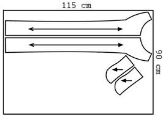
Şekil 1.2: Tela yerleşim planı
