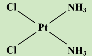
Cisplatin
