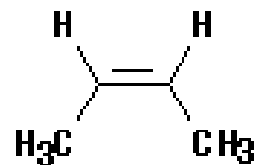
cis-2-butene (Z)-2-butene
