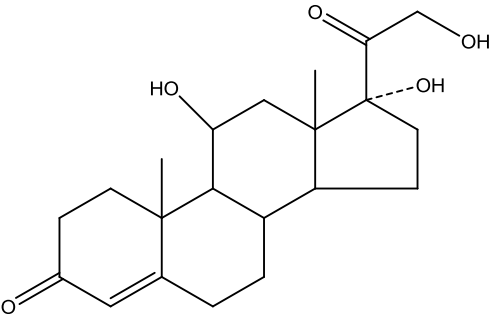
Hidrokortizon
