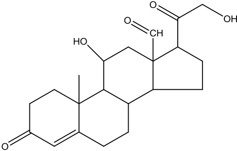
Aldosteron
