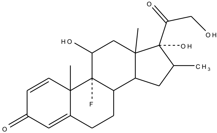
Betametazon
