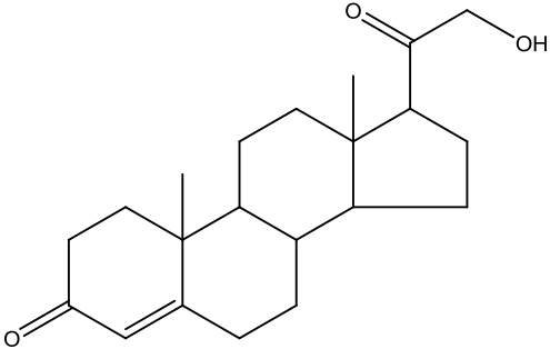
Dezoksikortikosteron
