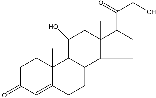
Kortikosteron
