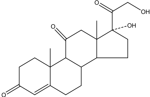
Kortizon
