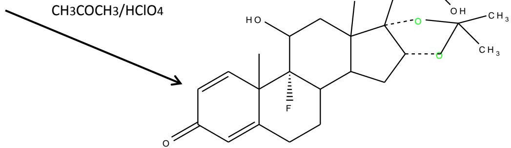
Triamsinolon asetonit
