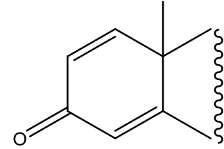
Prednizolon asetat
