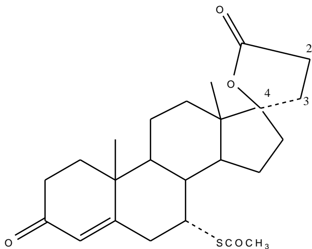
spironolakton
