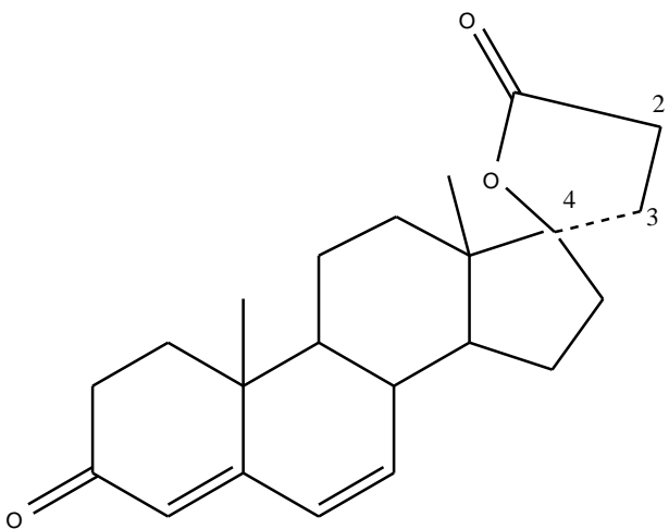
Kanrenon
