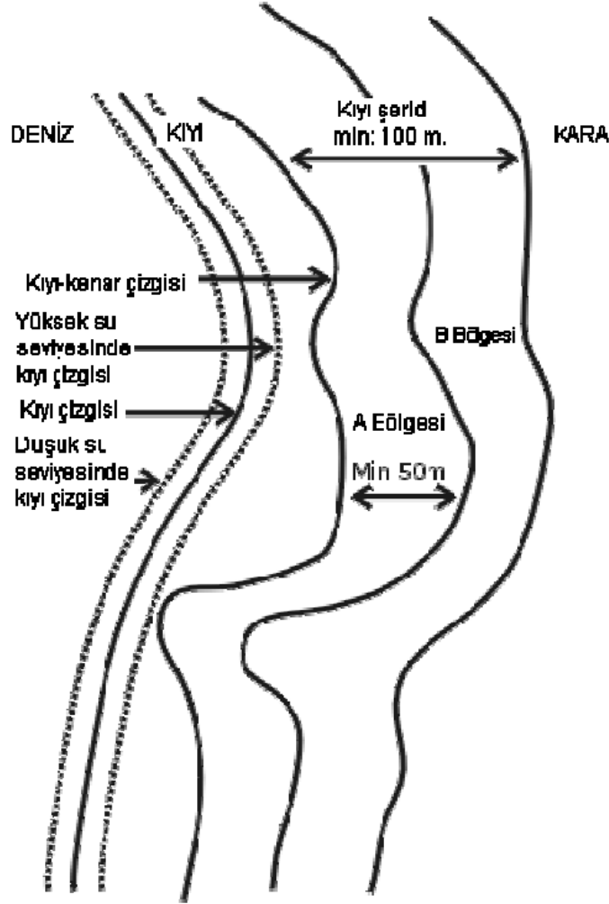
Şekil 2.2 Kıyılara ilişkin tanımlar (Özhan 1996)
