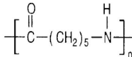
Poly(caprolactam) "Nylon"
